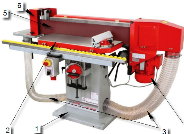
mașină de șlefuit cant: 1-batiu; 2-masă; 3-tuburi exhaustare; 4-motor; 5- bandă abrazivă; 6-apărător
