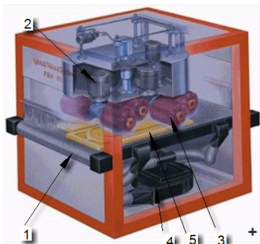
mașină de șlefuit cu perii: 1-bandă transportoare cauciucată; 2-motoare electrice; 3-perii rotative; 4-gură exhaustare; 5-piesă șlefuită
